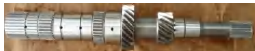
川崎驱动轴 Kawasaki Drive Shaft
